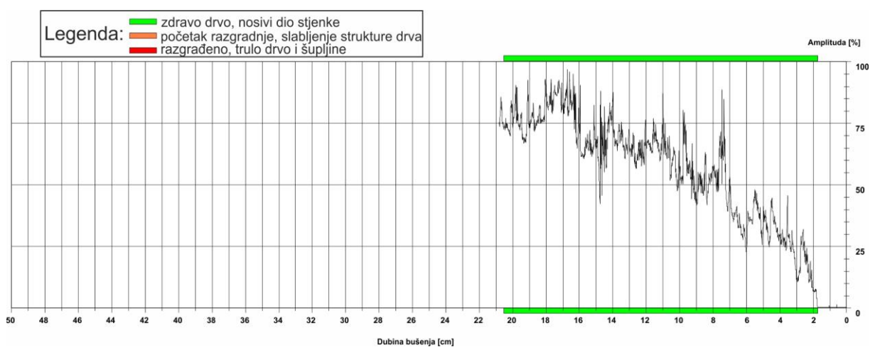
Slika 18: Rezistogram bušenja 5.1
