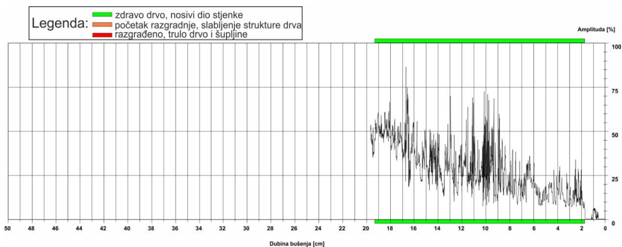
Slika 17: Rezistogram bušenja 5
