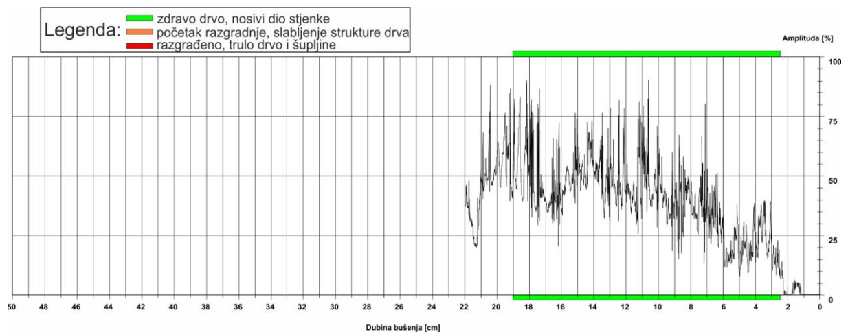
Slika 21: Rezistogram bušenja 6.1
