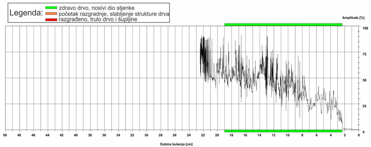
Slika 20: Rezistogram bušenja 6
