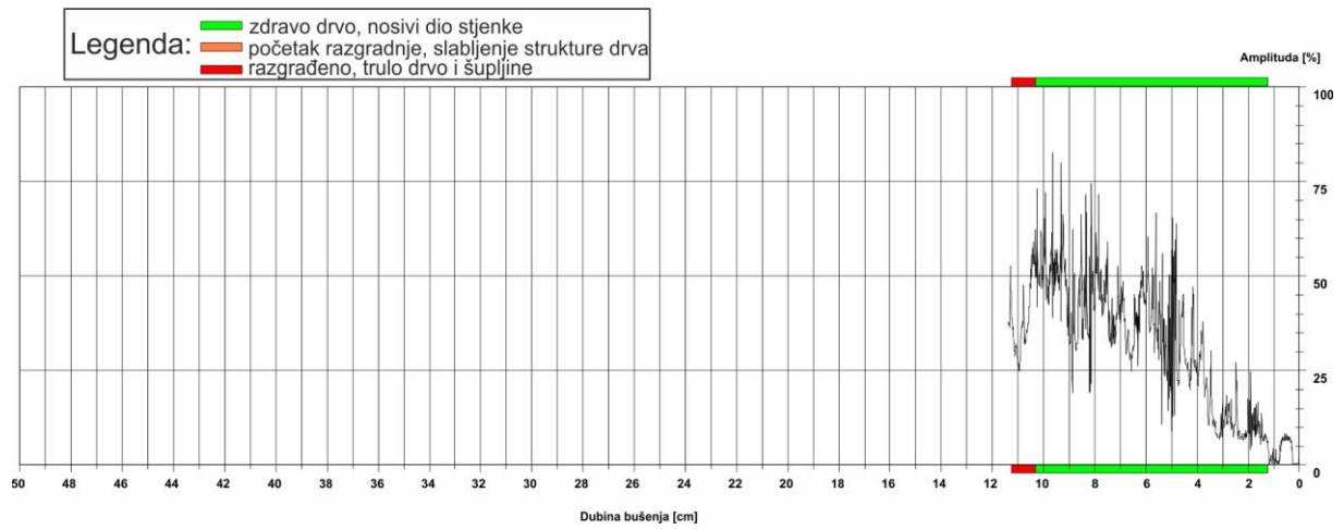
Slika 19: Rezistogram bušenja 7
