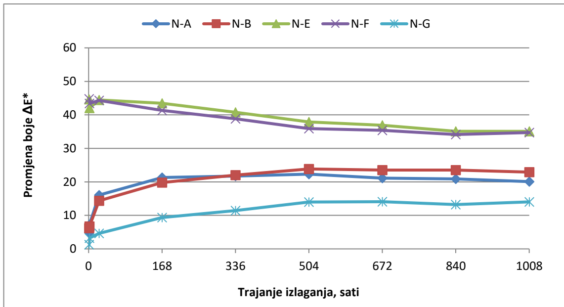
Slika 27. Promjena boje ( \Delta E^* ) nemodificiranih uzoraka premazanih emulzijama dobivenih IN SITU postupkom i uzoraka premazanog čistim poliakrilatom bez \text{TiO}_2
