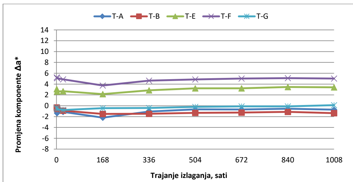
Slika 18. Promjena koordinata a^* ( \Delta a^* ) toplinski modificiranih uzoraka premazanih emulzijama dobivenih IN SITU postupkom i uzoraka premazanog čistim poliakrilatom bez TiO_2
