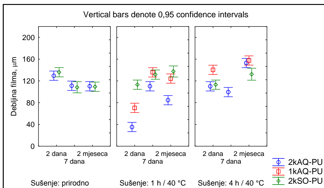
Slika 31. Utjecaj vrste, trajanja sušenja i trajanja kondicioniranja na debljinu slobodnog filma lakova na bazi poliuretana (2kAQ-PU: dvokomponentni vodeni lak, 1kAQ-PU: jednokomponentni vodeni lak, 2kSO-PU: dvokomponentni otapalni lak)
