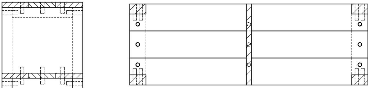
Presjek B-B
