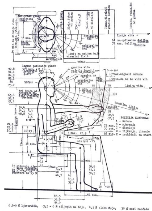
Slika 7 Antropometrijske (dinamičke) dimenzije za mušku populaciju u sjedećem položaju
