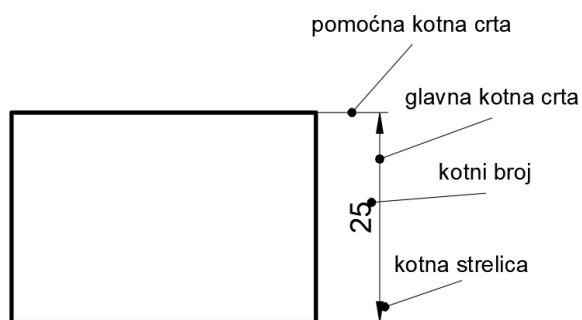
Slika 4.1 Elementi kote
