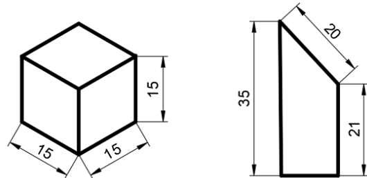
Slika 4.6 Kotiranje vertikalnih i kosih crta
