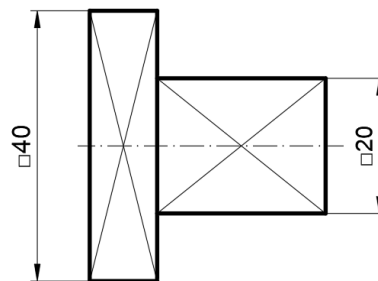
Slika 4.16 Kotiranje kvadratičnoga presjeka
