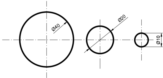
Slika 4.14 Kotiranje promjera
