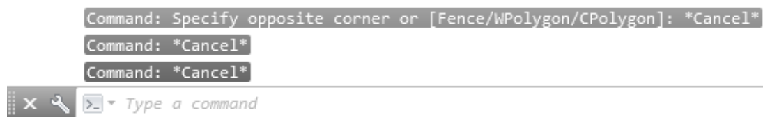
Slika 7.11 Naredbeni redak
