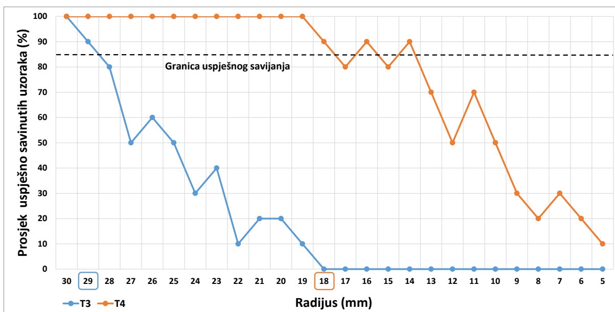
Slika 53: Graf usporedbe testiranja T3 (nepareni) i T4 (pareni), uzorci: 1 mm, tangentialna tekstura
