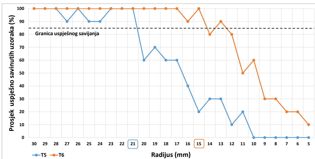
Slika 54: Graf usporedbe testiranja T5 (nepareni) i T6 (pareni), uzorci: 0,6 mm, radialna tekstura
