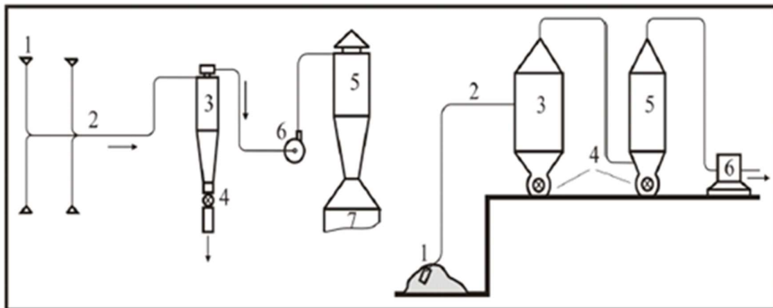
Slika 5. Uspisni zračni konvejer
