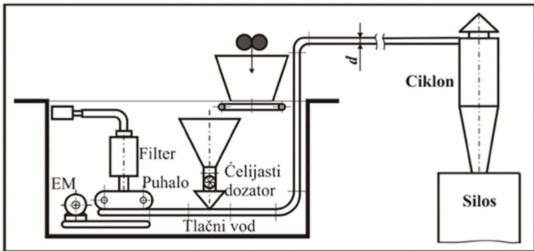
Slika 7. Tlačni sustav
