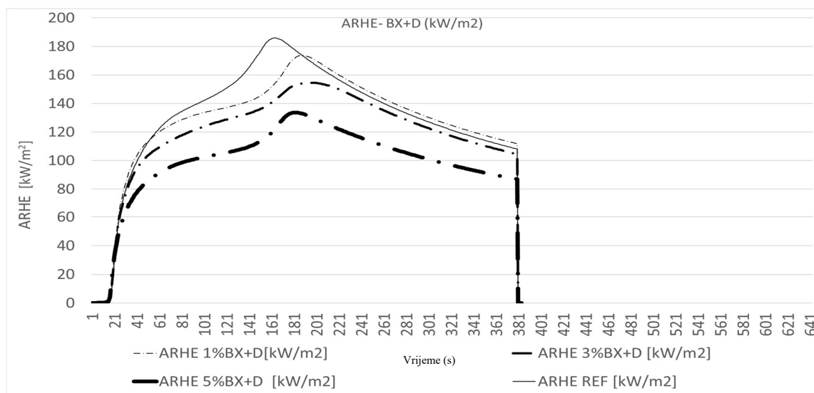
Slika 41. Grafički prikaz iznosa ARHE (prosječna brzina emisije topline) u \text{kW/m}^2 za vrijeme ispitivanja BX+D uzoraka izmjenjenih konusnim kalorimetrom
