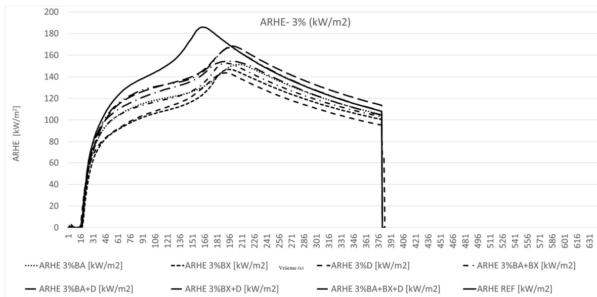
Slika 44. Grafički prikaz iznosa ARHE (prosječna brzina emisije topline) u \text{kW/m}^2 za vrijeme ispitivanja uzoraka s 3 % koncentracijom izmjerenih konusnim kalorimetrom
