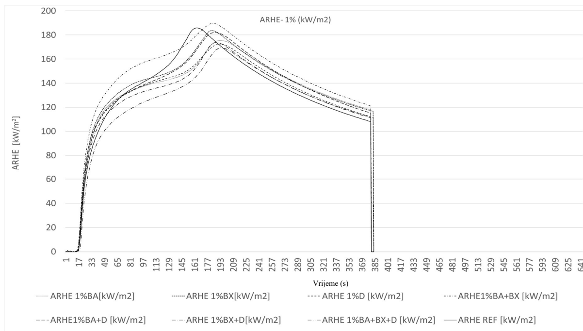
Slika 43. Grafički prikaz iznosa ARHE (prosječna brzina emisije topline) u \text{kW/m}^2 za vrijeme ispitivanja uzoraka s 1 % koncentracijom izmjerenih konusnim kalorimetrom
