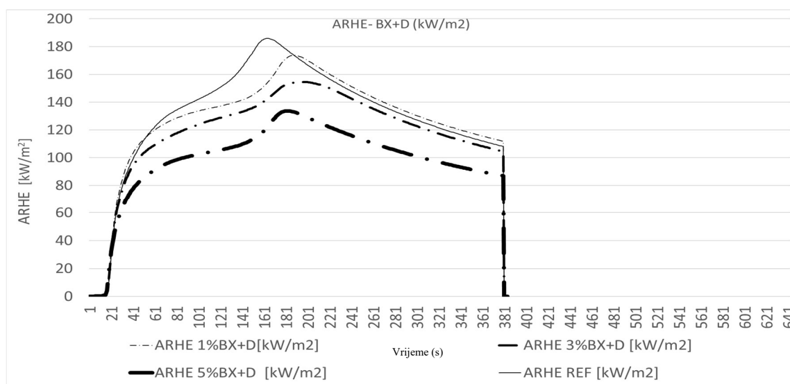
Slika 41. Grafički prikaz iznosa ARHE (prosječna brzina emisije topline) u kW/m 2 za vrijeme ispitivanja BX+D uzoraka izmjerenih konusnim kalorimetrom
