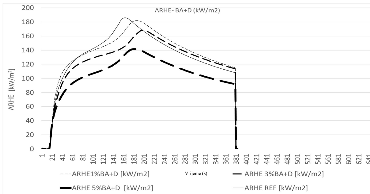
Slika 40. Grafički prikaz iznosa ARHE (prosječna brzina emisije topline) u kW/m 2 za vrijeme ispitivanja BA+D uzoraka izmjerenih konusnim kalorimetrom
