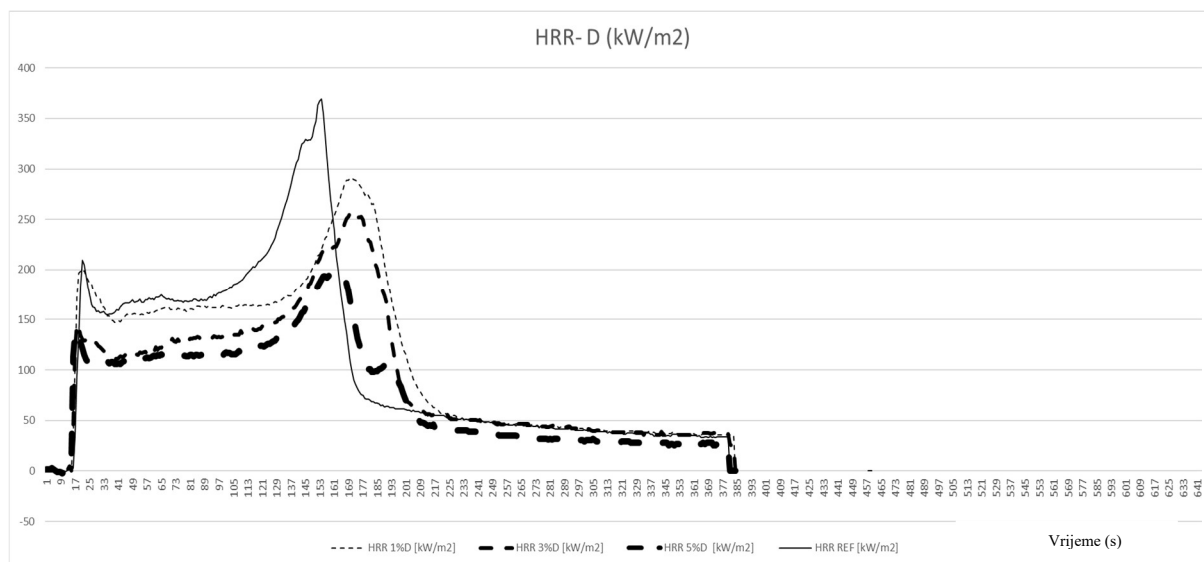
Slika 49. Grafički prikaz iznosa HRR (brzina oslobađanja topline) u kW/m 2 za vrijeme ispitivanja D uzoraka izmjenjenih konusnim kalorimetrom
