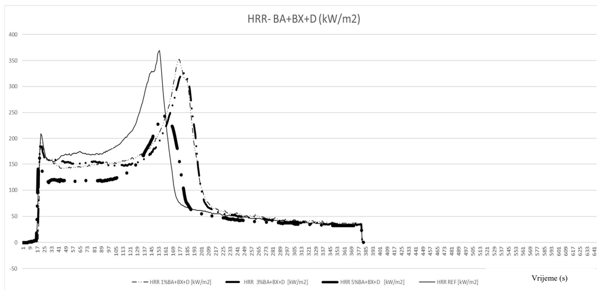
Slika 53. Grafički prikaz iznosa HRR (brzina oslobađanja topline) u \text{kW/m}^2 za vrijeme ispitivanja BA+BX+D uzoraka izmjenjenih konusnim kalorimetrom
