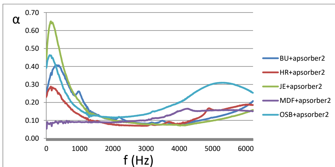
Slika 48. Usporedba uzoraka s apsorberom 2 pri visokim frekvencijama
