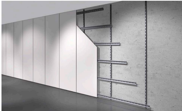
Slika 15. Membranski apsorber sa metalnim nosačima (Egger acoustic katalog 2016)
