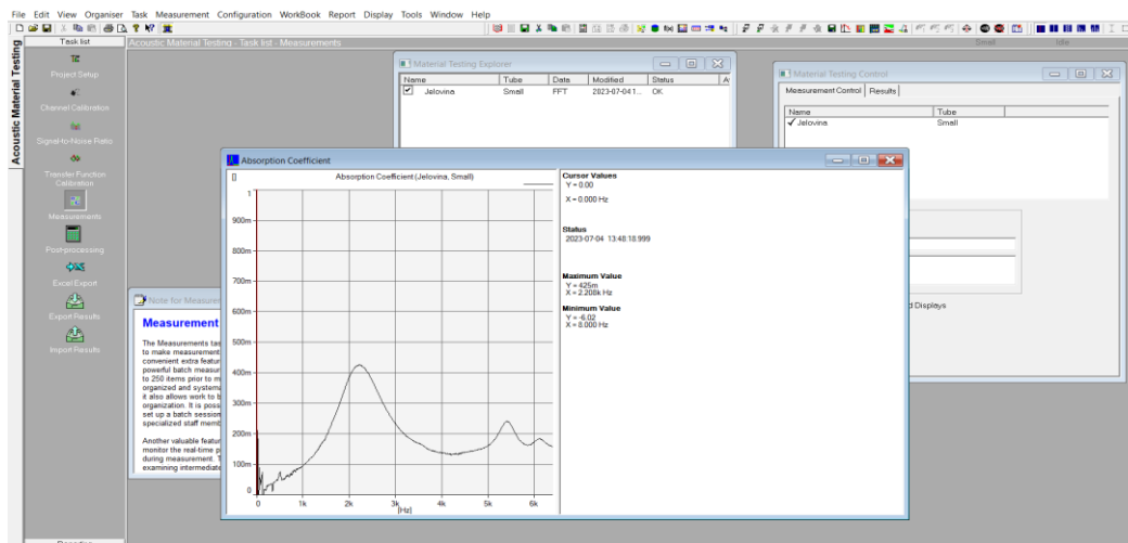
Slika 30. Program PULSE
