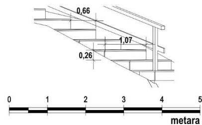
Slika 36. Detalji stepenica
