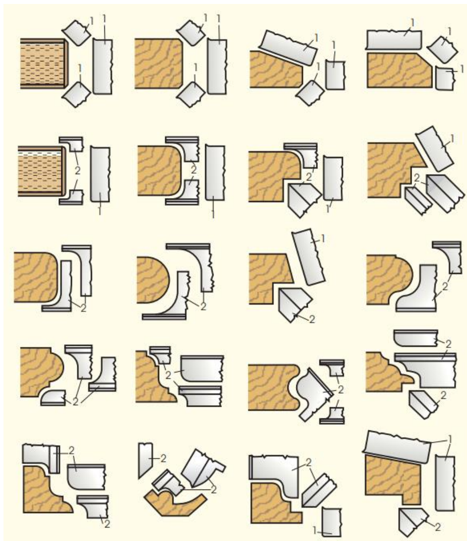
Slika 10. Brušenje profila (Jaić i Živanović-Trbojević, 2000.)
