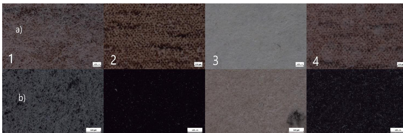
Slika 31. Usporedba površine tretiranih uzoraka Compact ploče kiselinom kroz 24 sata a) uzorci s dekorom hrasta b) uzorci s crnim dekorom (1- sulfatna kiselina, 2- octena kiselina, 3- nitratna kiselina 4- solna kiselina)
