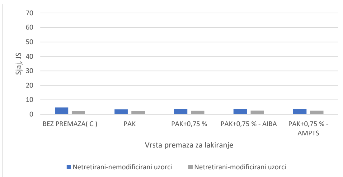
Slika 25. Sjaj površine nemodificiranih i modificiranih prije premazivanja
