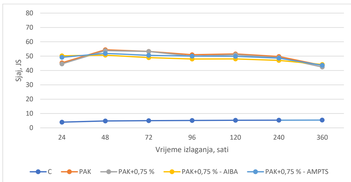
Slika 27. Sjaj površine nemodificiranih uzoraka tijekom izlaganja
