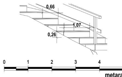
Slika 36. Detalji stepenica
