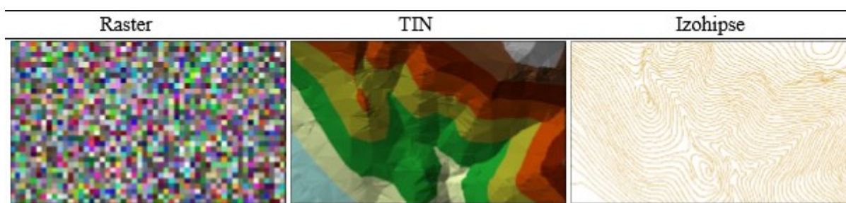
Slika 8 Osnovne strukture za predstavljanje površina u digitalnom obliku (Izvor: Šiljeg, A., 2013)
