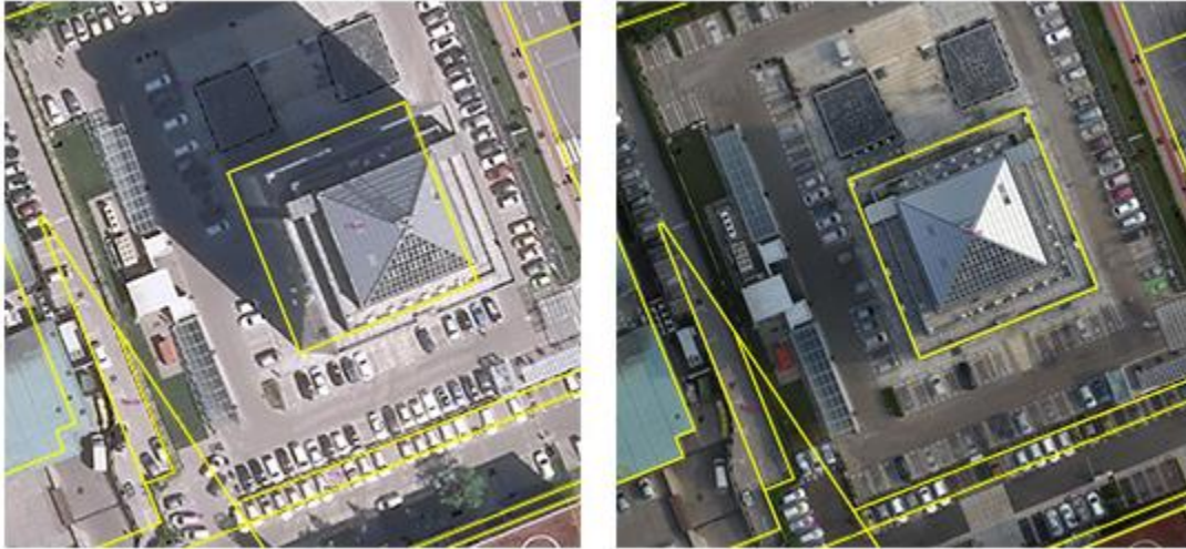
Slika 3. Primjer običnog ortofota (lijevo) i pravog ortofota (desno) ( https://www.geavis.si/en/2015/09/how-are-true-orthophoto-mosaics-made/ )
