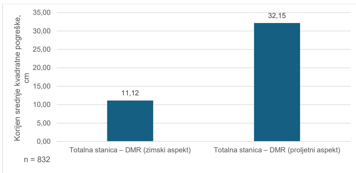
Slika 28. Korijen srednje kvadratne pogreške (nekorigirane) z koordinata terenskih točaka između referentne metode i DMR-ova (zimski i proljetni aspekt)
