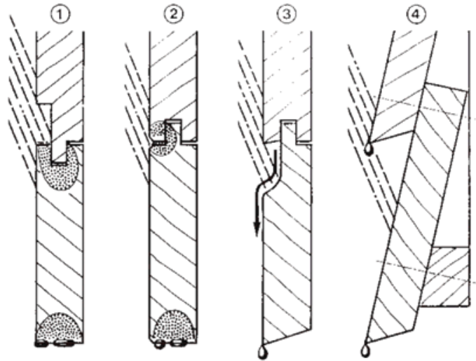
Slika 7. Primjeri dobre i loše konstrukcijske zaštite pročelja (erlinger-holzbau.at).
