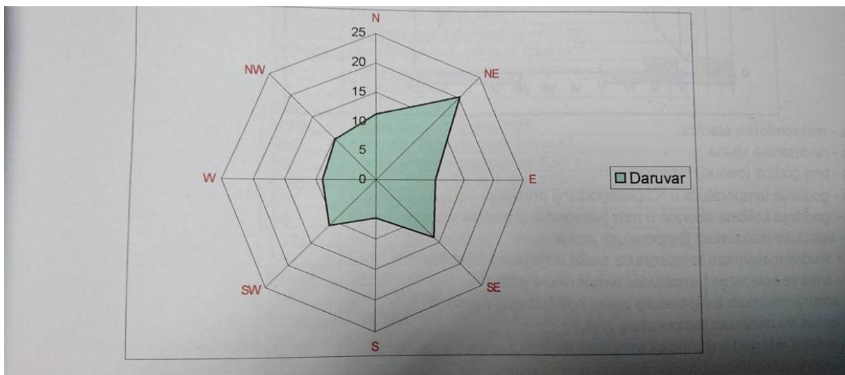
Slika 2. Ruža vjetrova
