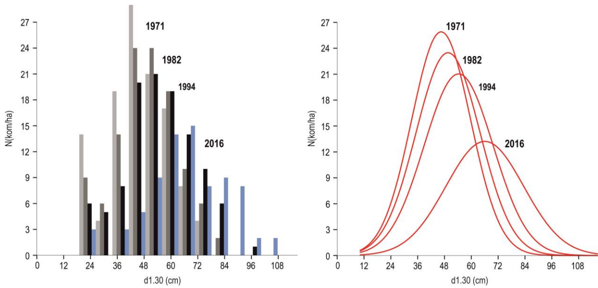
Slika 9. Izmjerene (lijevo) i izjednačene (desno) distribucije prsnih promjera za hrast lužnjak na pokusnoj plohi prema godinama inventure
