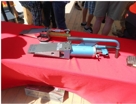
Slika 5. Mehanički klin za obaranje stabala
