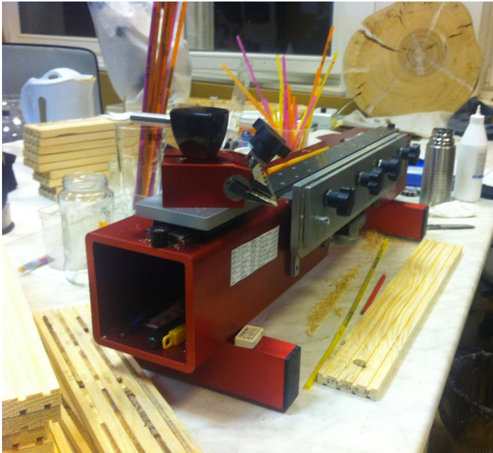
Slika 18. Dendroekološki laboratorij s kliznim mikrotomom (foto: Krešimir Begović)
