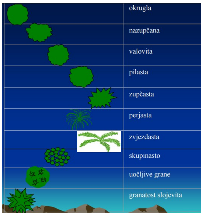
Slika 3. Oblici krošanja
