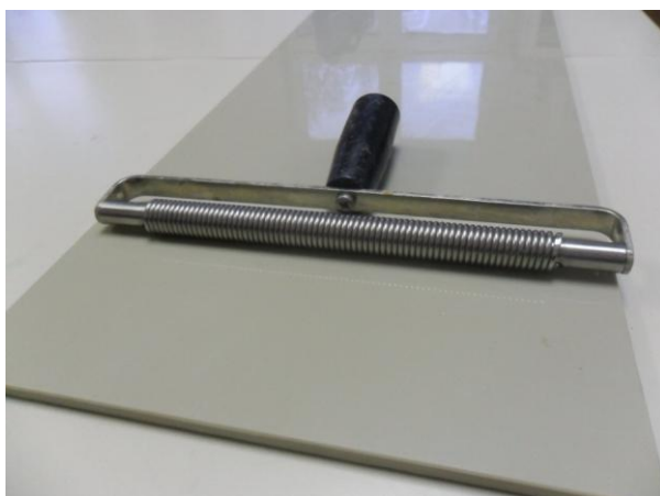
Slika 10. Nanošenje premaza spiralnim aplikatorom na polipropilensku ploču
