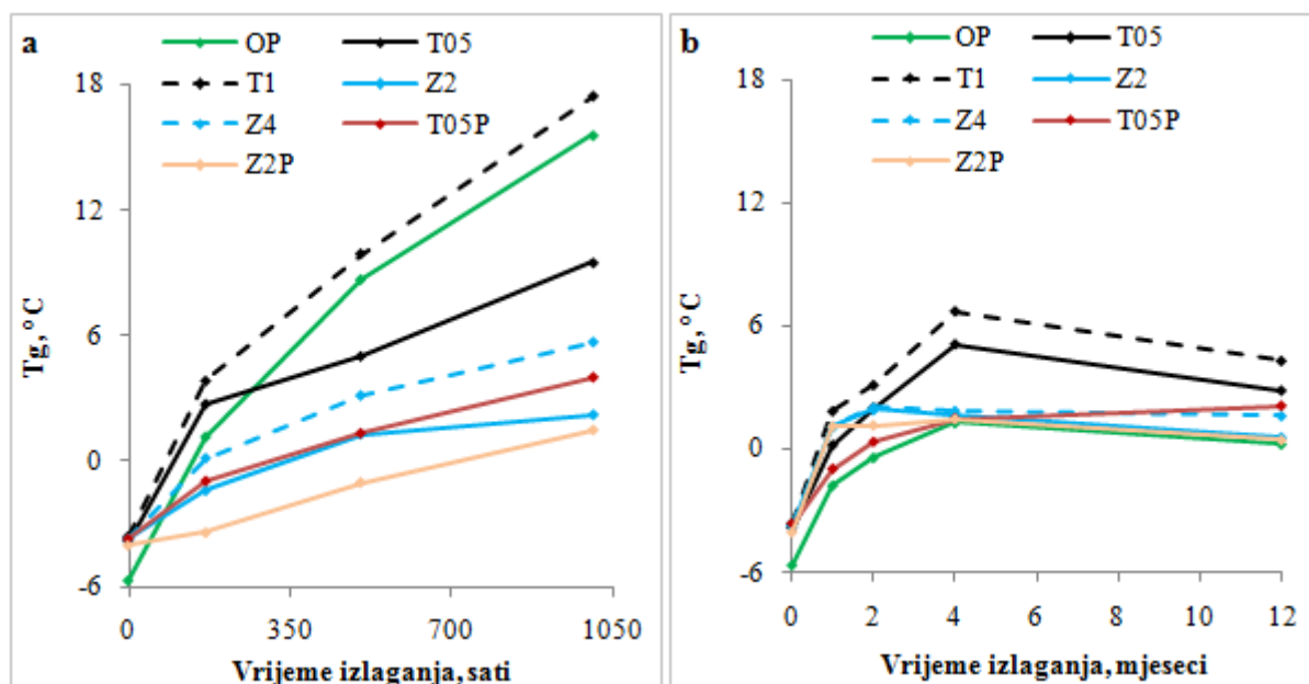
Slika 43. Promjena staklišta ( T_g ) premaza tijekom ubrzanog (a) i prirodnog (b) izlaganja
