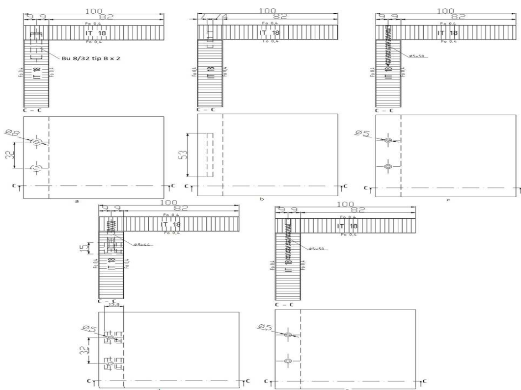
Slika 13. Prikaz uzoraka sastavljenih pomoću: a) moždanika, b) eliptičnog umetka, c) vijka za drvo, d) svornjaka sa zaokretnim klinom i e) "Conformat" vijka (Župčić i suradnici, 2012.) 39
