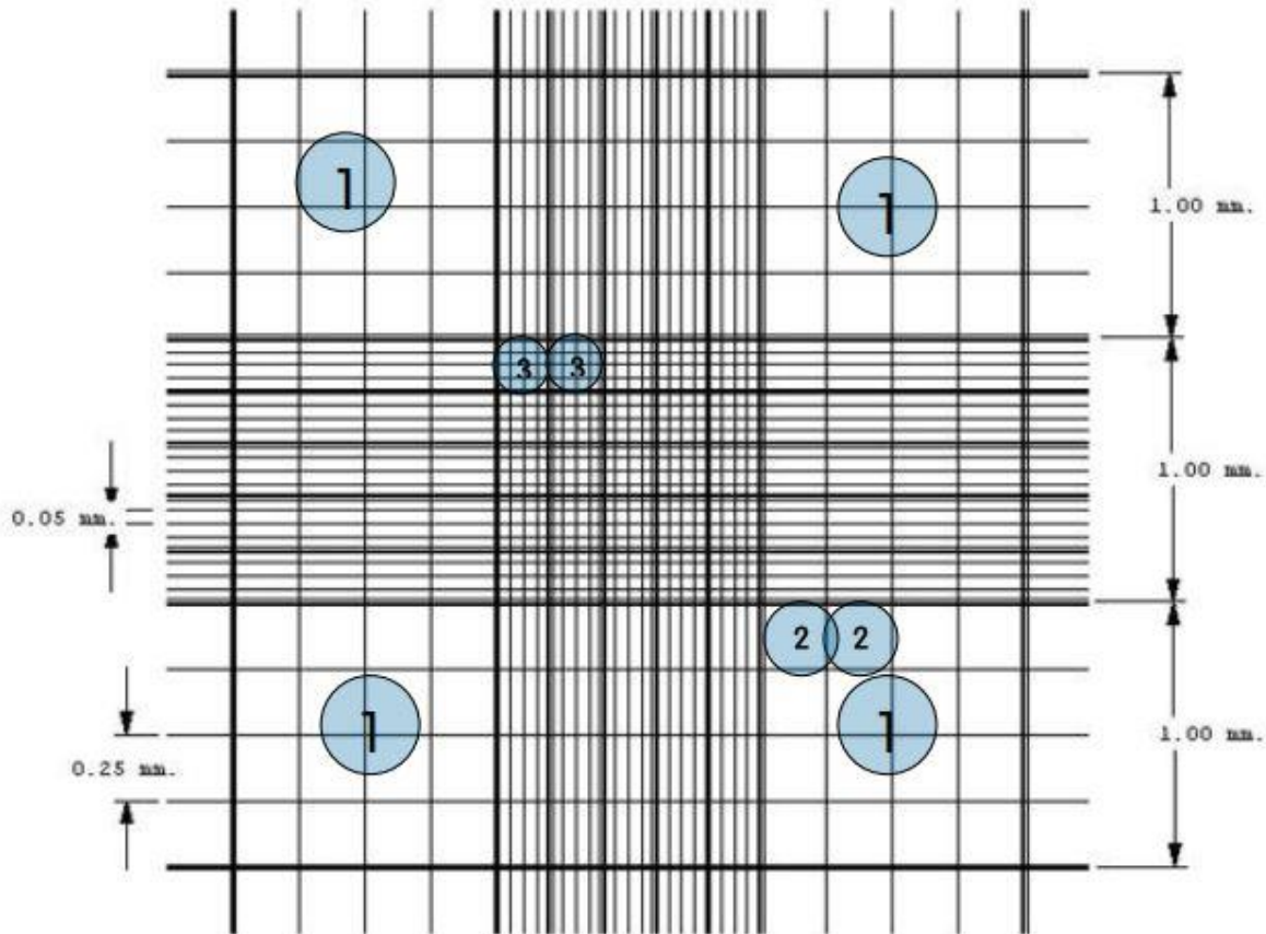
Slika 23. Mreža za brojanje spora u Neubauer komorici Figure 23. Neubauer chamber grid for counting spores
