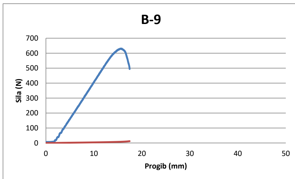
Slika 16. Prikaz dijagrama napreznja za uzorak B-9
