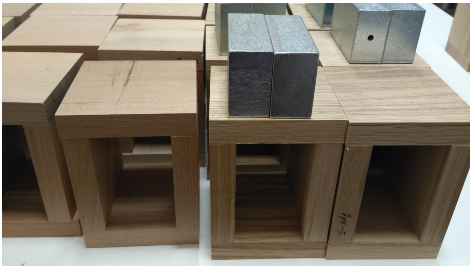
Slika 5. Prešanje uzoraka
